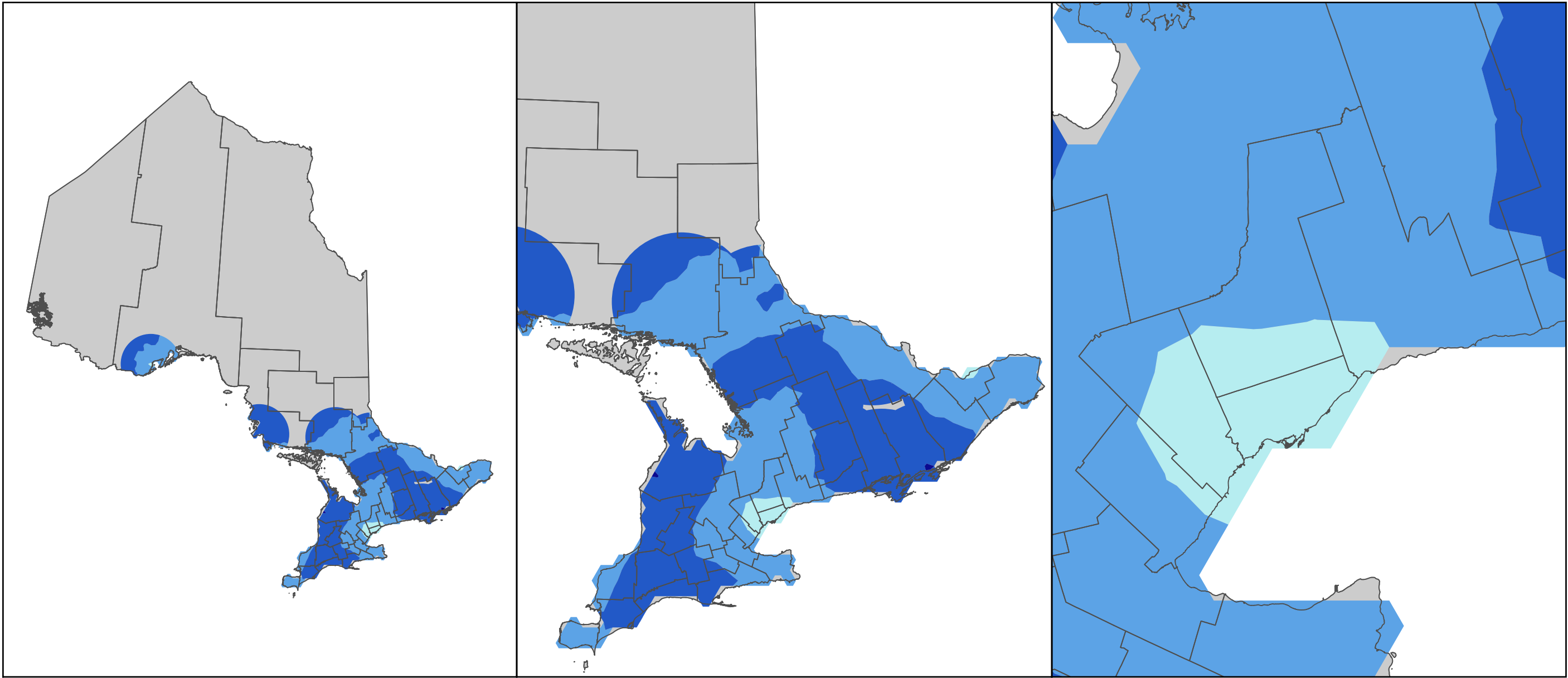
Ozone (parts per billion)
